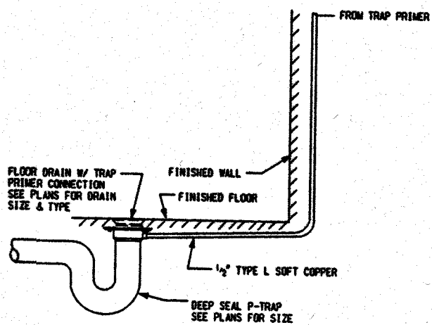
TRAP PRIMER DETAIL SCALE: NONE
